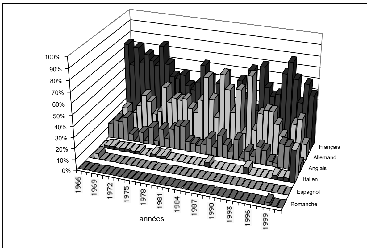
Fig. 3. Langues rédactionnelles
